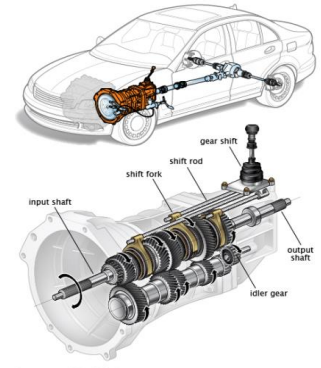
Hộp số bằng tay
